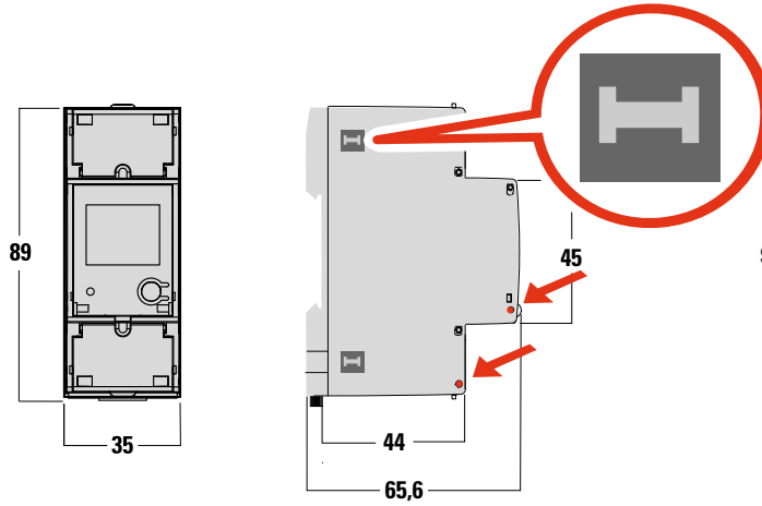
Plombierbares Gehäuse und Klemmenabdeckung Sealed housing and sealable terminal block
