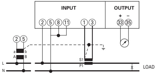
Wechselstromnetz Single-phase
