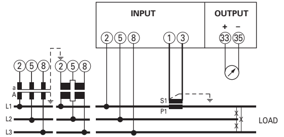
3-Leiter Drehstromnetz, gleich belastet Three-phase 3-wire, balanced load
